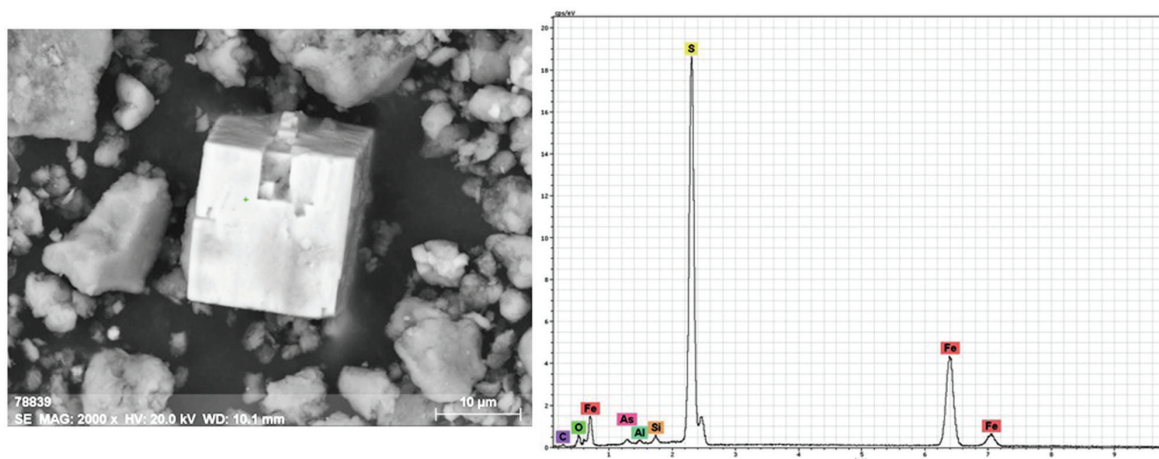
Рис. 4. Снимок в режиме обратно рассеянных электронов и энергодисперсионный спектр кубического кристалла пирита FeS_2 (масс. %: S – 45; Fe – 44) / Fig. 4. Snapshot in the backscattered electron mode and the energy-dispersive spectrum of a cubic crystal of pyrite FeS_2 (wt. %: S – 45; Fe – 44)
